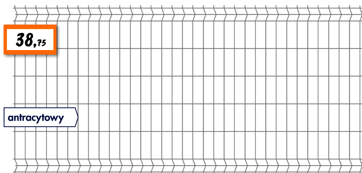
Panel 3D wym. 2,5x1,23 m, oczko 75x200 mm, drut Ø 3,2 mm nr ref. 20268220
