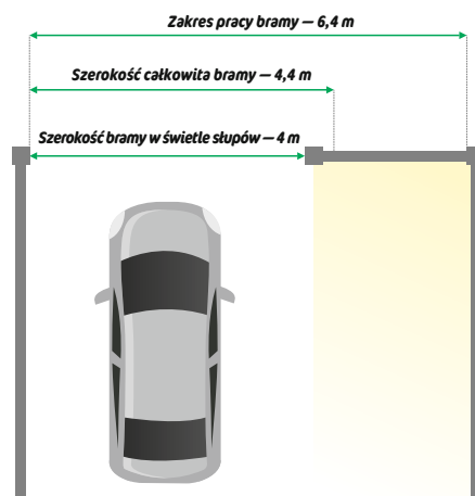
Brama segmentowa
